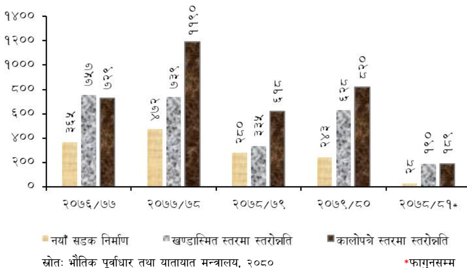
चाई १०(क): पछिल्लो ५ वर्षको सडक निर्माणको स्थिति (किलोमिटर)
