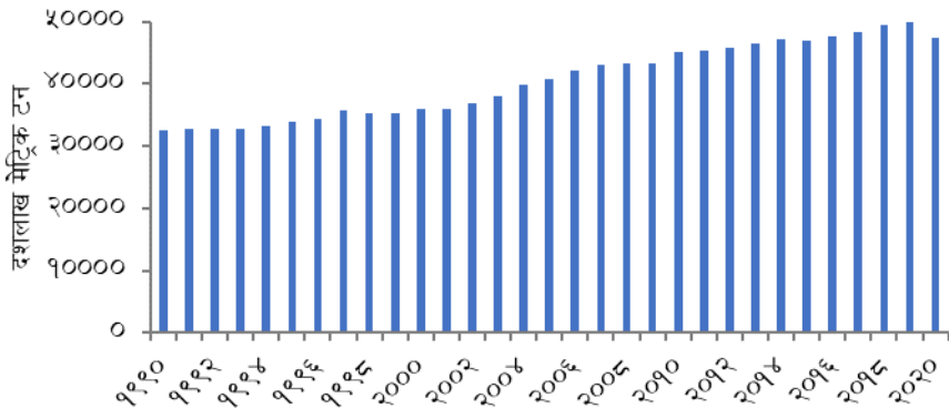
चार्ट १४(क): विश्वको हरितगृह ग्यास उत्सर्जनको प्रवृत्ति
