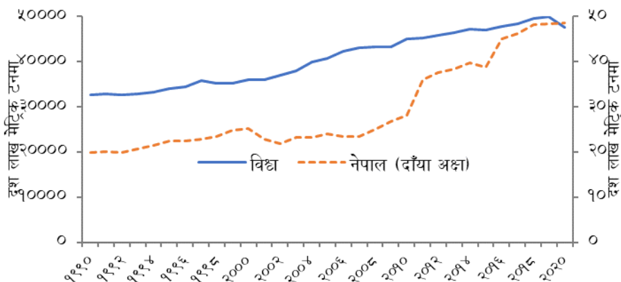
चार्ट १४(ख): नेपाल र विश्वको हरितगृह ग्यास उत्सर्जनको प्रवृत्ति
