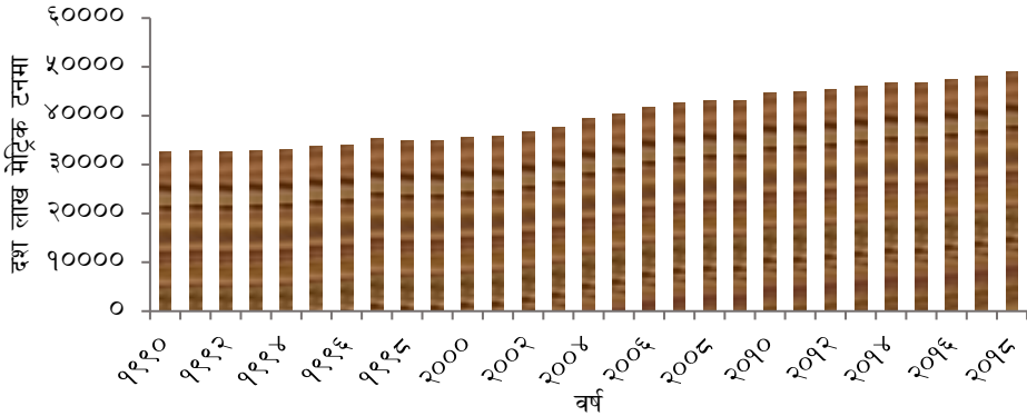
चार्ट १६(क): विश्वको हरित गृह ग्यास उत्सर्जनको प्रवृत्ति (सन् १९९० देखि २०१८)
